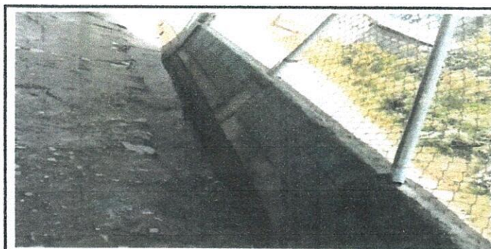
Foto 5: Reparación de Muro de Contención con reforzamiento con cuneta y drenes, lado sur del centro educativo
