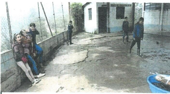
Foto 4: Reparación de Muro de Contención con reforzamiento con cuneta y drenes, lado sur del centro educativo
